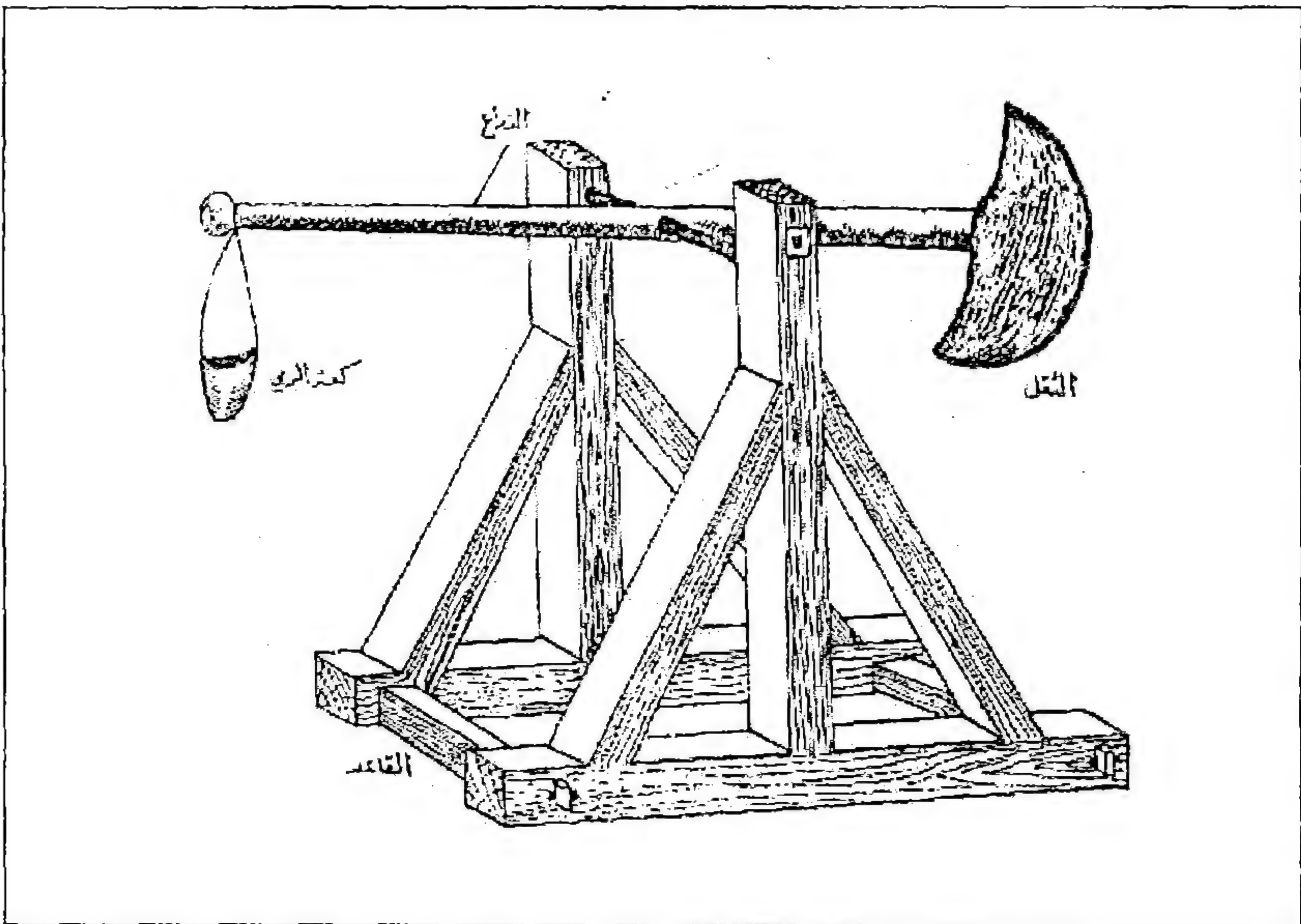
الشكل رقم (٢٩) المحتوى (رسم لألة المنجنيق)
